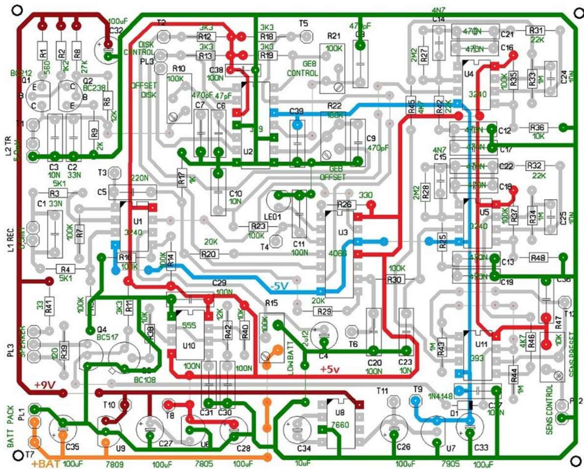
Рис. 26(2): Размещение шин питания на печатной плате.
