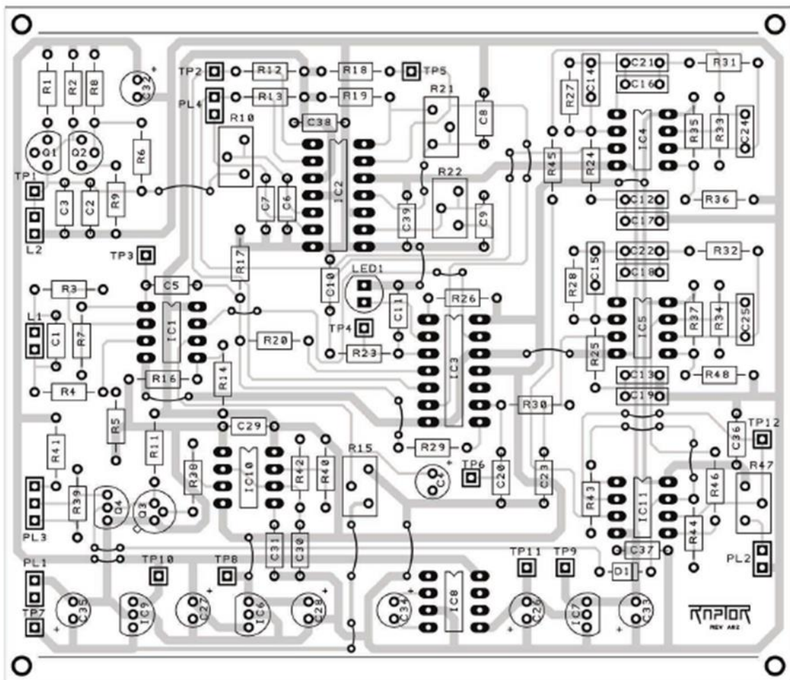
Рис. 26: Размещение деталей на печатной плате.
